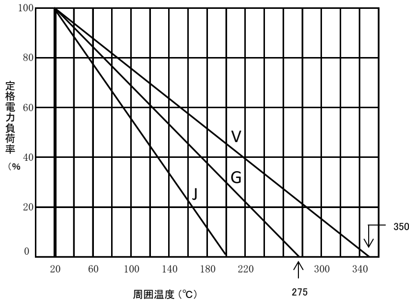
図1 負荷電力低減曲線
