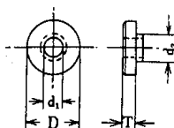
セラミック スペーサー
